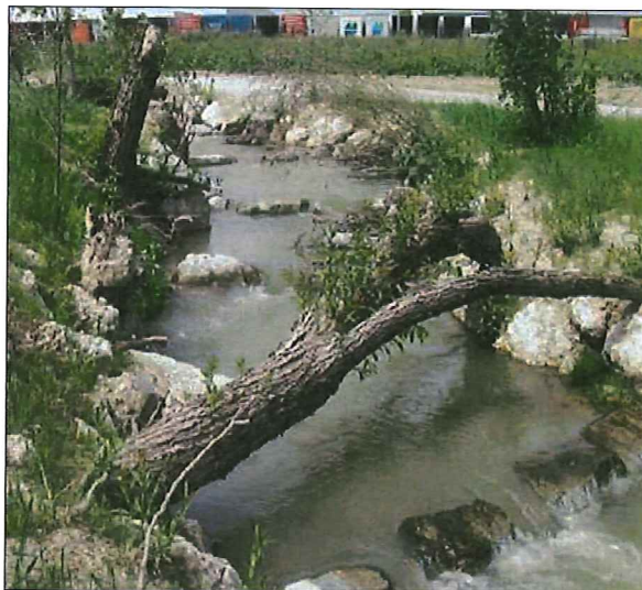
Slika 2: Primer izvedbe izrazito neporavnanih utrjenih brežin s skalami samicami in kamni (privzeto iz Grundlagen für einen österreichischen Leitfaden zum Bau von Fischaufstiegshilfen (FAHs). Bundesministerium für Land- und Forstwirtschaft, Umwelt und Wasserwirtschaft, Wien, 2011).
