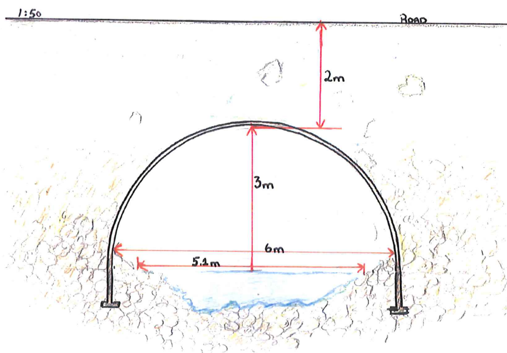
Slika 1: Prikaz izvedbe za ribe ustreznega cestnega prepusta z izvedbo sonaravno oblikovanega grobega dna struge (privzeto iz Culvert Design for the Protection of Fishery Resources, Report , T. Tavčar, T. Pittman in A. Trogrlič, 2007).
